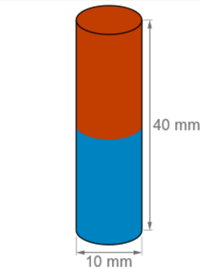
Måltegning · alle mål i mm
