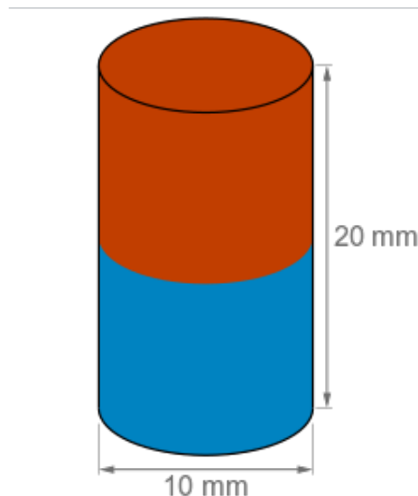
Måltegning · alle mål i mm
