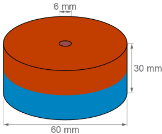
Måltegning · alle mål i mm
