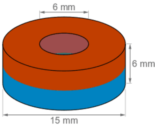
Måltegning · alle mål i mm
