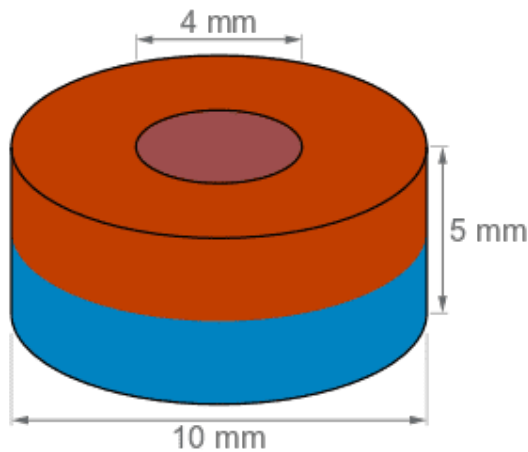
Måltegning · alle mål i mm
