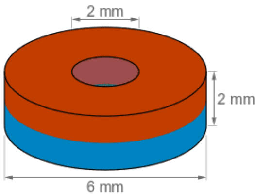
Måltegning · alle mål i mm
