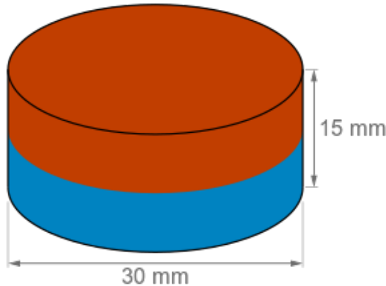
Måltegning · alle mål i mm
