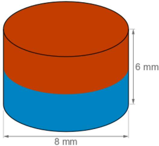
Måltegning · alle mål i mm
