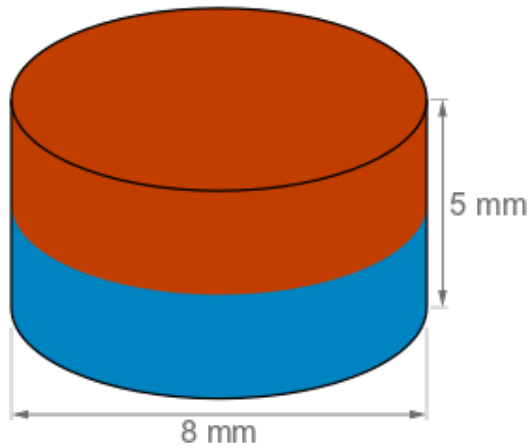
Måltekening · alle mål i mm
