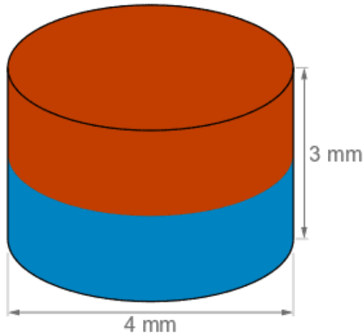
Måltekening · alle mål i mm
